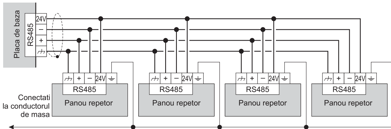
Figure 17 Cablarea Repetoarelor
