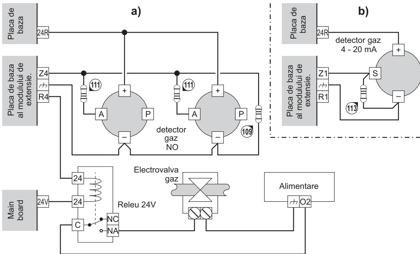
Figura 16 Cablarea detectoarei de Gaz cu iesire Normal Deschis(a) si un detector Gaz 4-20 mA (b): 109) 3900 ohm, 1/4W EOL (oranj-alb-rosu-auriu); 111) rezistor 680 ohm; 113) rezistor 470 ohm, 2W
